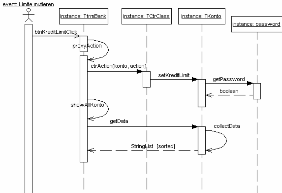
Abb. 5: Sequencediagramm
